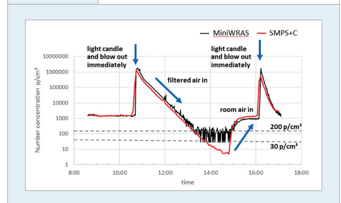
Zeitlicher Verlauf der MiniWRAS Gesamtpartikelanzahlkonzentration im Vergleich zum GRIMM SMPS+C mit Kerzen als Partikelquelle
